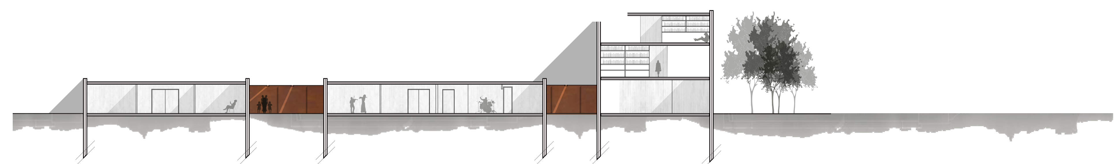
COUPE BB' 1:200 BIBLIOTHEQUE - ECOLE - LOGES
