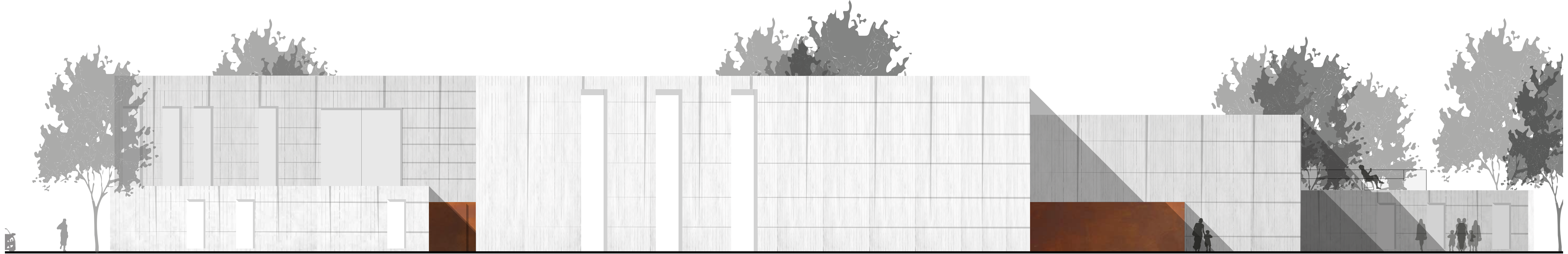
FACADE NORD / VUE DU TRAM 1:100
